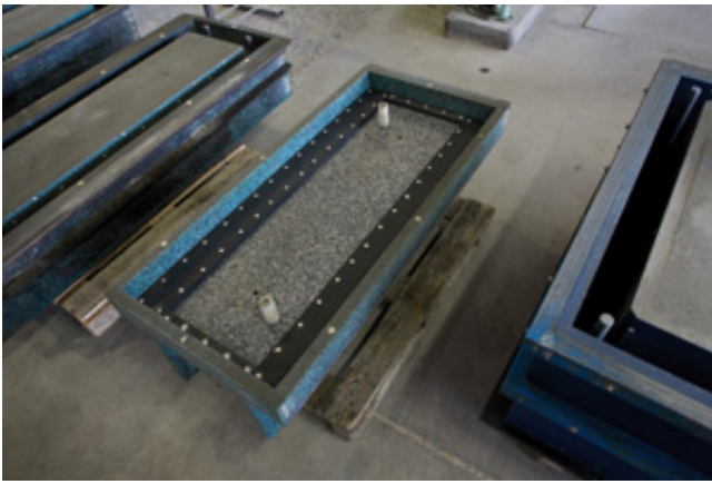
Kunststoffform zur Herstellung von Betonwaren
