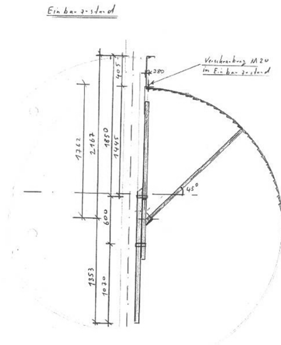
Skizze Einbauzustand (Darstellung aus statischer Berechnung)
